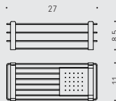
B9632 Angolaring Porta oggetti da doccia e vasca con ripiano inox Basket for shower and bath with stainless steel shelf
