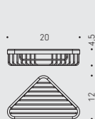
B2732 Angolare semplice Single corner basket
