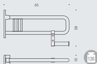
B9729 Appoggio ribaltabile con portarotolo Folding support with paper holder
