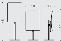
B9753 Specchio ingranditore (3x) d'appoggio regolabile in altezza Standing magnifying mirror (3 times), adjustable in height
