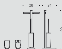
B9108 Piantana (Base 24x14 cm) con doppio porta rotolo e porta scopino Floor standing column with double paper holder and brush holder
