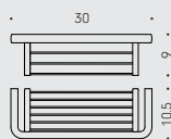
B6232 Porta oggetti da doccia e vasca Basket for shower and bath
