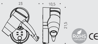
B9970 Asciugacapelli da parete con presa universale per rasoio 110/220V Automatic wall hair dryer with universal shaver socket 110/220V
