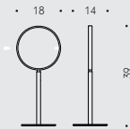
B9752 Specchio ingranditore (3x) d'appoggio Standing magnifying mirror (3 times)
