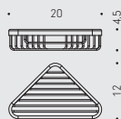
B2732 Basic Angolare semplice Single corner basket
