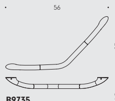
B9735 Maniglione da vasca Bath grab-bar complies with UNI 11064:2003
