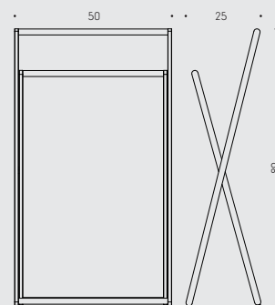
B9737 Cavalletto porta salviette H.89 Rack
