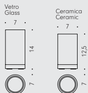
B5241 Porta bicchiere d'appoggio Standing glass holder
